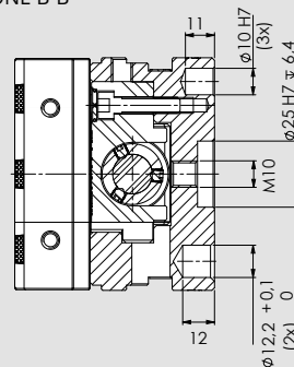
SEZIONE B-B
