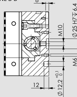
SEZIONE B-B
