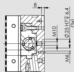
SEZIONE B-B
