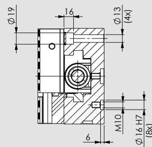
SEZIONE B-B
