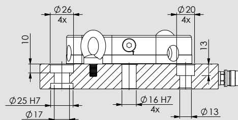
SEZIONE C-C
